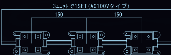
■製品寸法
