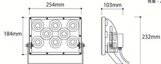
商品詳細図 質量 : 2.38kg
