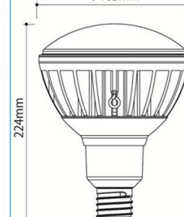
E39 LED 電球 45W/70W
