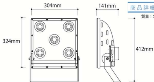
商品詳細図 質量 : 5.64kg
