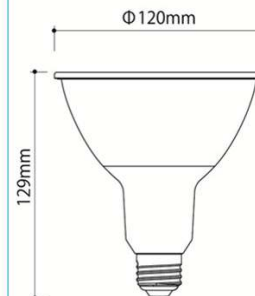
ビーム球 16W
