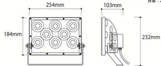
商品詳細図 質量 : 2.38kg
