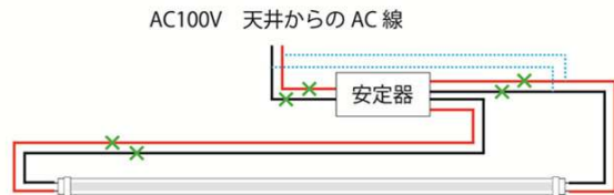
結線図
