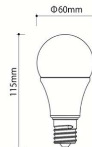
E26 白熱球タイプ
