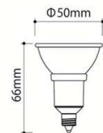
ミニクリプトンビーム球 4W
