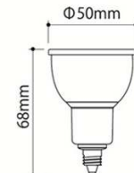
ミニクリプトンビーム球 5W
